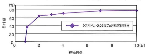
■ピレスロイド薬剤各種の経過日数に伴うチャバネゴキブリ感受性系統の致死率(2反復合計、雄20頭、雌20頭)
